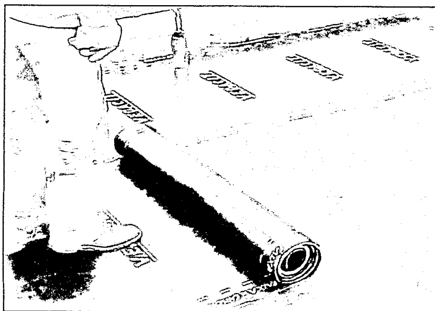
Figura 2 – Imagem do sistema de aplicação de impermeabilização em manta asfáltica.
