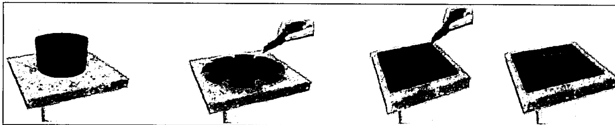
Figura 6 – Imagens esquemáticas de aplicação de manta asfáltica em ralo.
