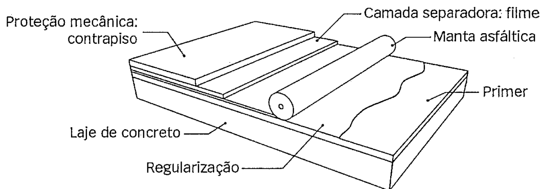
Figura 3 – Desenho esquemático de camadas de sistema de impermeabilização.
