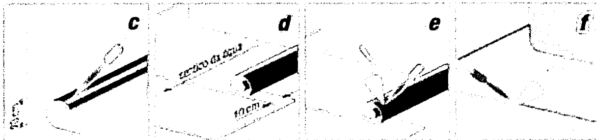
Figura 4 – Desenho esquemático de aplicação da manta asfáltica.
